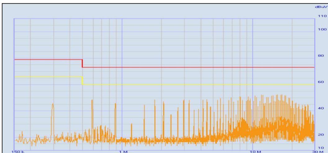
电源模块基础切换带宽 260 kHz.
