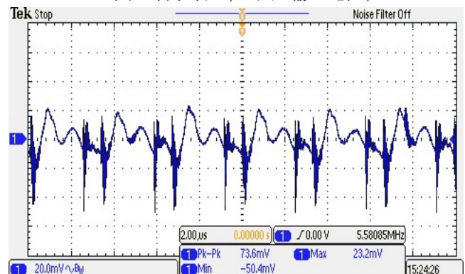
图 8: 输出电压纹波与噪声(满载). (典型输入, 于输出端加 1uF MLCC 陶瓷电容)
