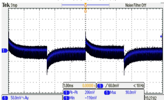
图 7: 进阶负载的输出变化 (典型输入, 于 50~70%的 \Delta I_o/\Delta t = 1A/\mu S 输出电流)
