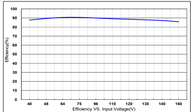
图 2: 效率值 VS 输入电压(满载)
