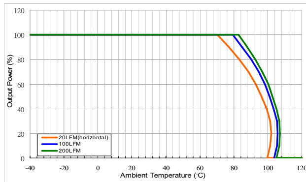
图 3: 环境温度 VS 输出效率降曲线
