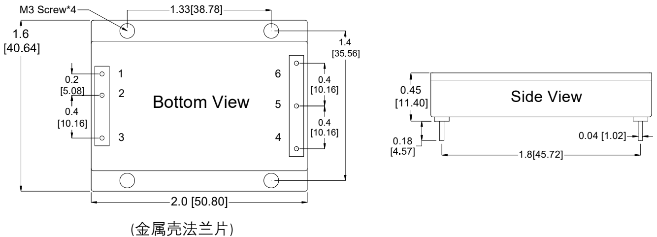
尺寸图 - B (金属壳法兰片)
