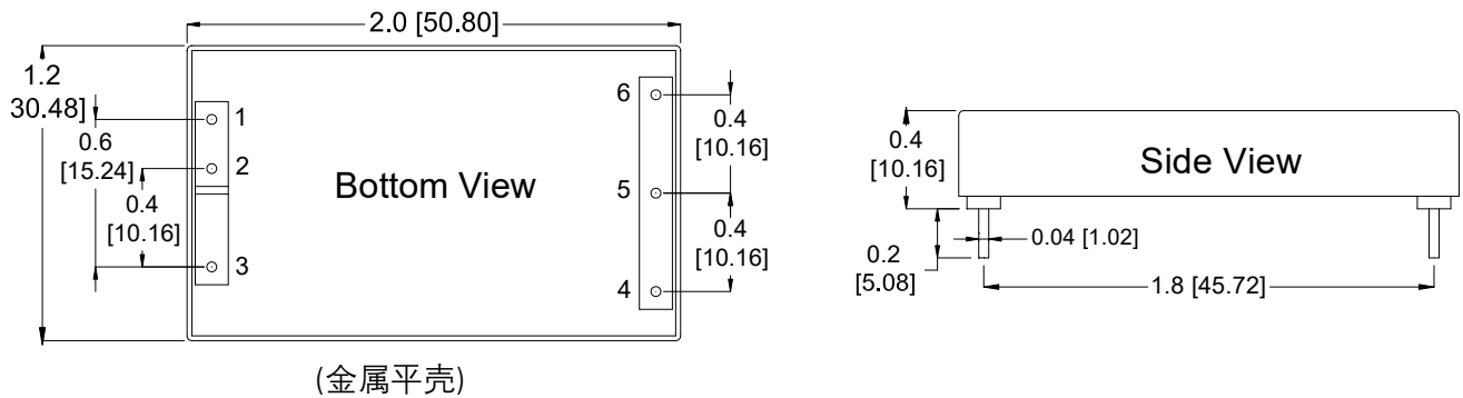
尺寸图 - P 金属切槽壳
