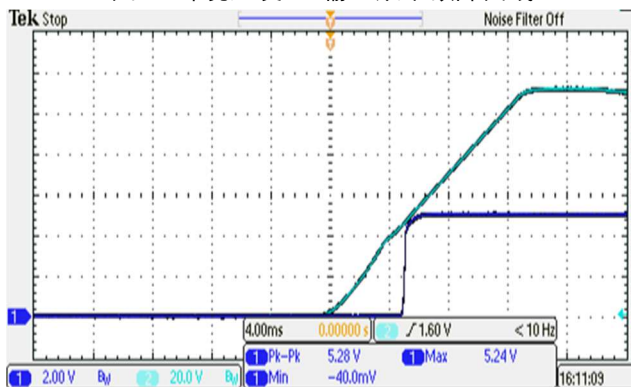
图 5: CH1 = 输出电压, CH3 = 额定输入电压 典型启动波形(满载)
