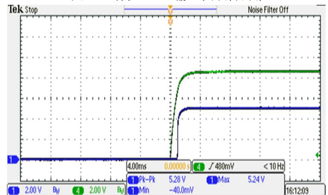
图 6: CH1 = 输出电压, CH3 = 远程遥控电压 典型启动波形(已设定输入电压)
